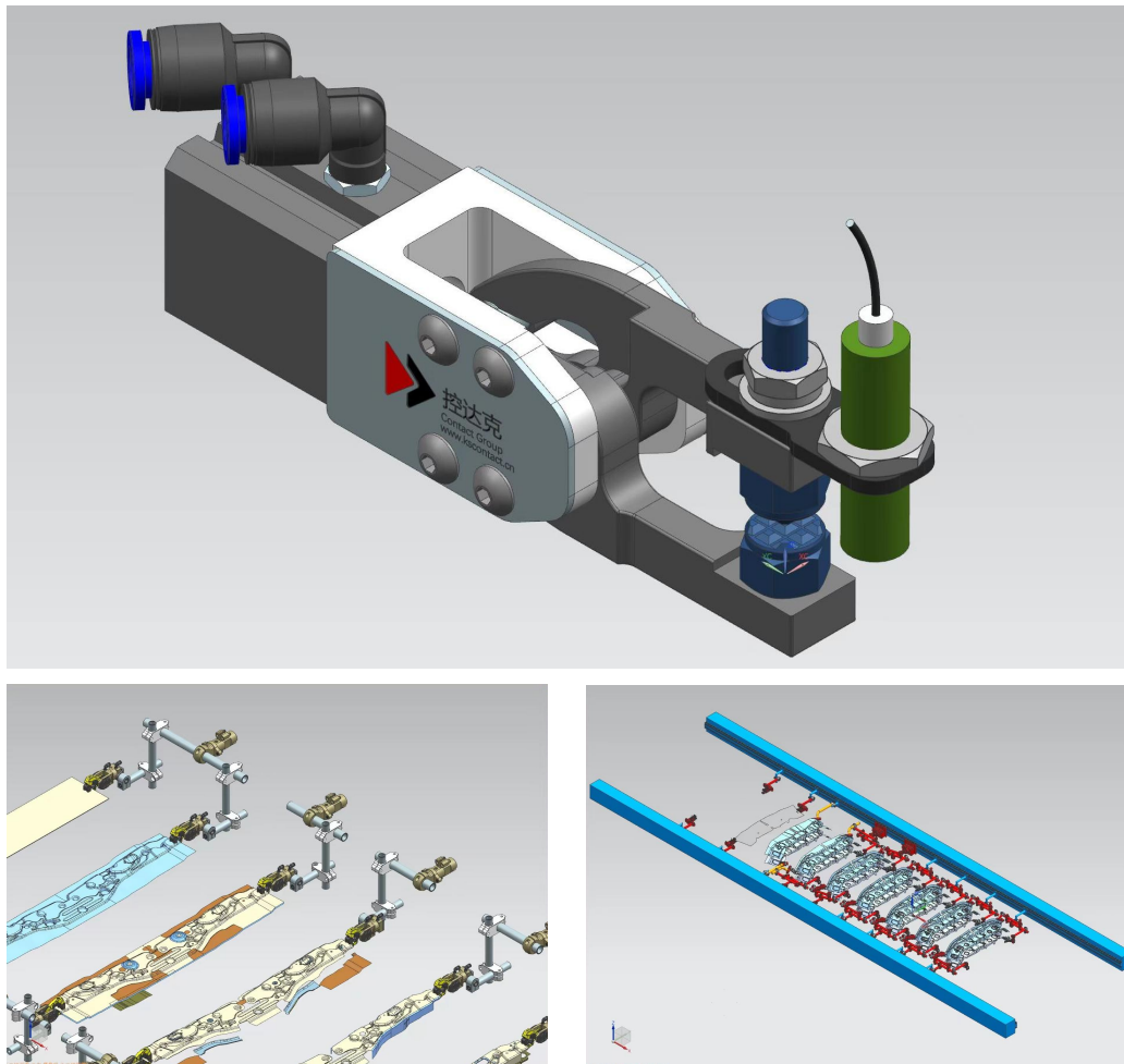
气 动 夹 钳
